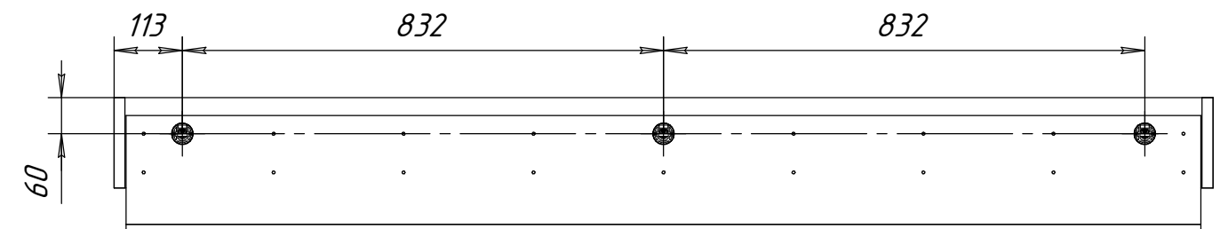
Полка 52.029.00.00
