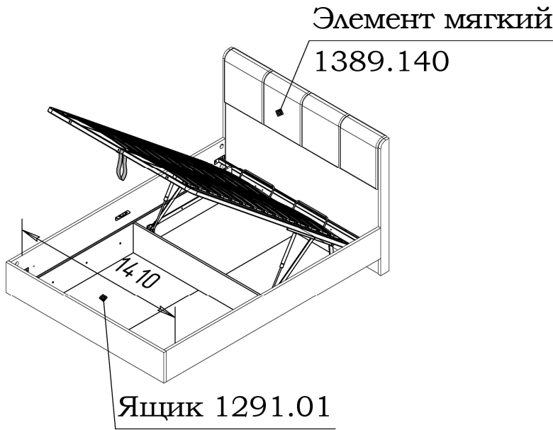
Кровать 82.200.00.00-01
