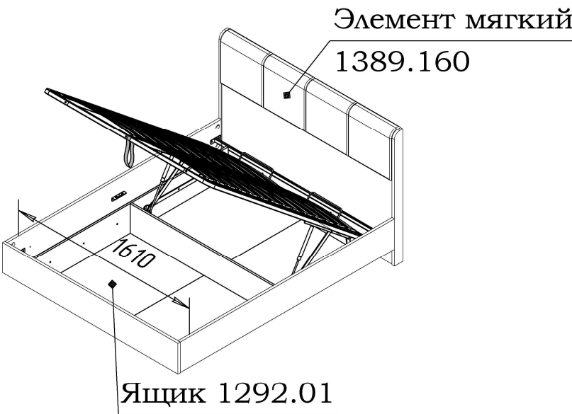
Кровать 82.201.00.00-01
