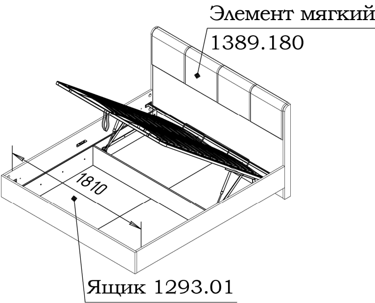
Кровать 82.202.00.00-01
