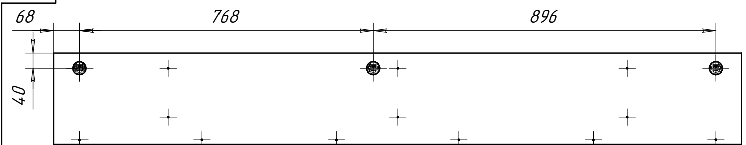
Схема полки 51.343.00.00 (вид сзади)
