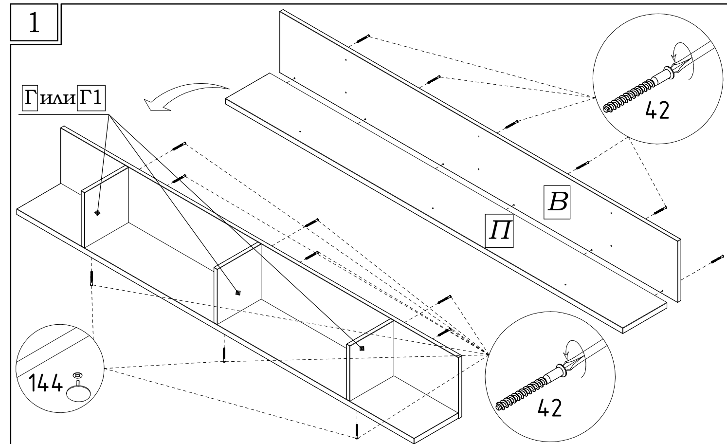
Схема полки 51.343.00.00 (вид сзади)
