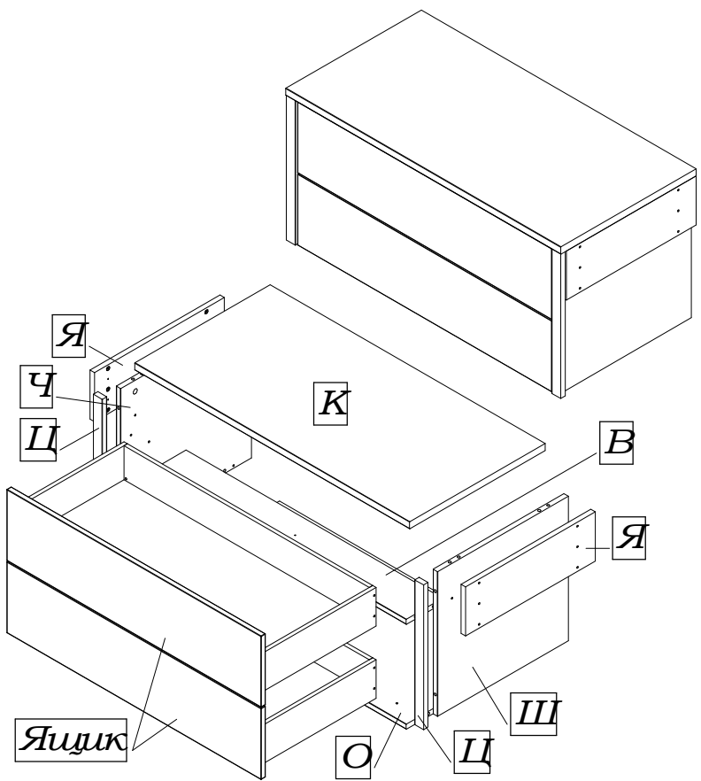
Тумба 21.304.00.00.00 (-01)
