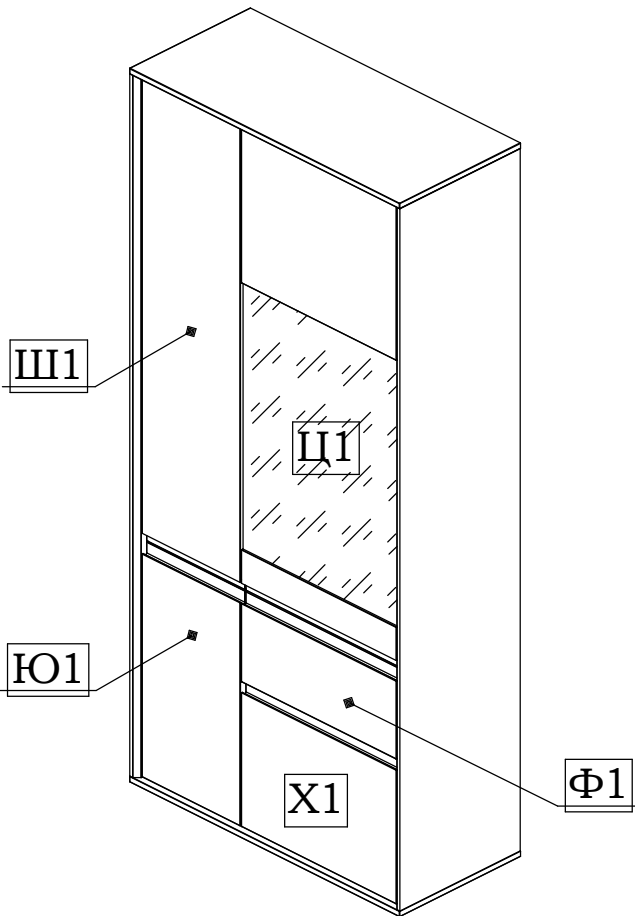
Шкаф 56.025.00.00.00.00-01
