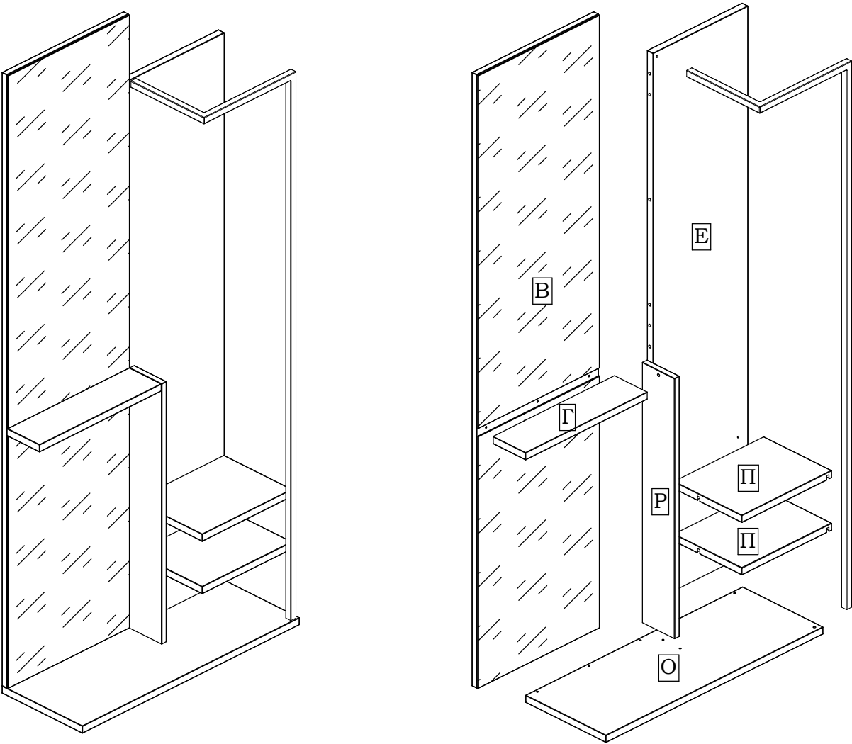
Вешалка 64.060.00.00.00
