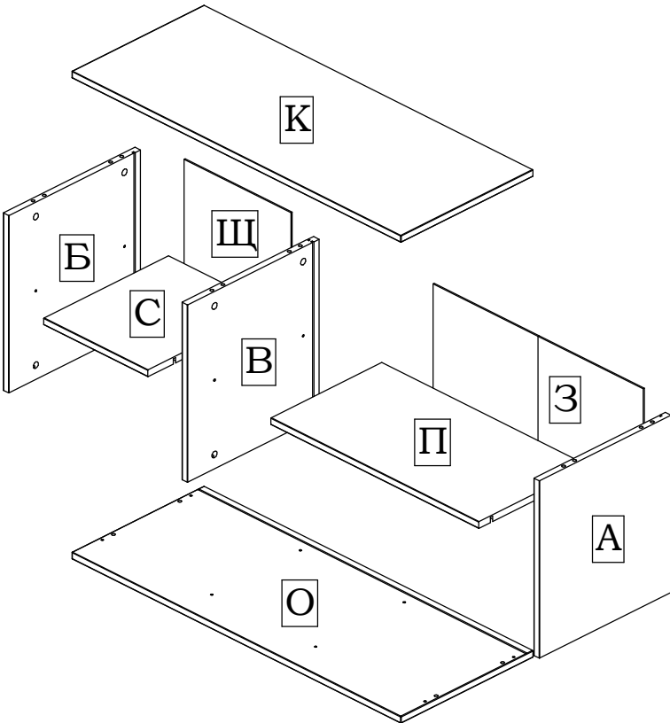
Вариант сборки
