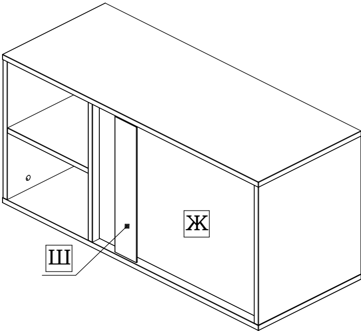
Вариант сборки
