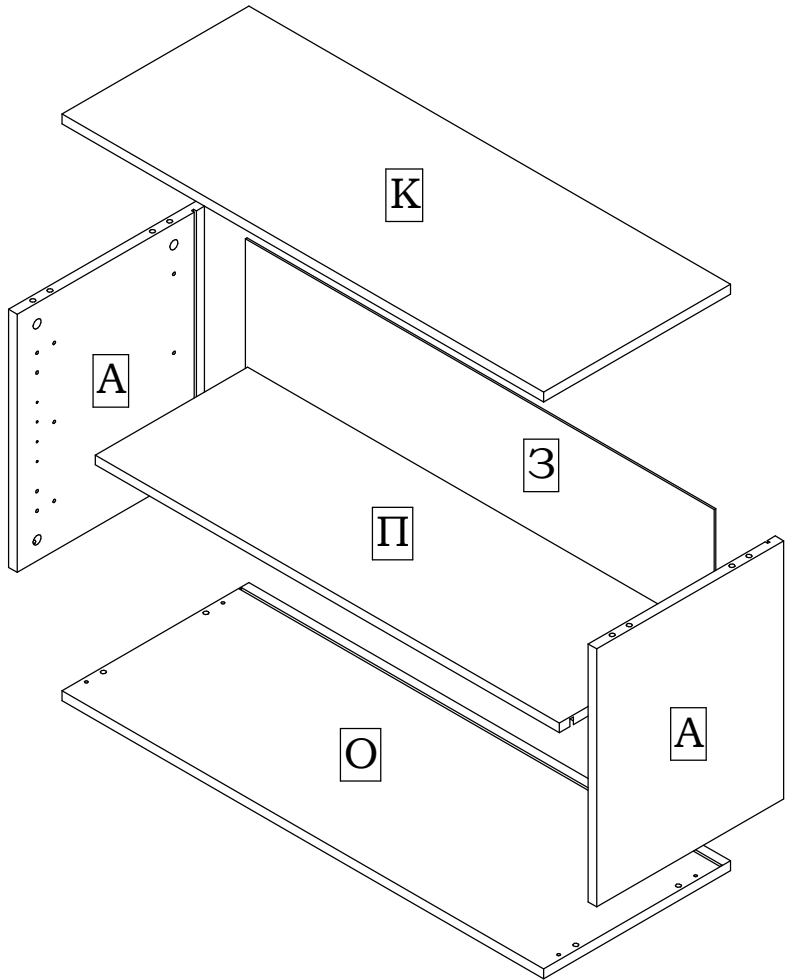
Комплект корпуса
