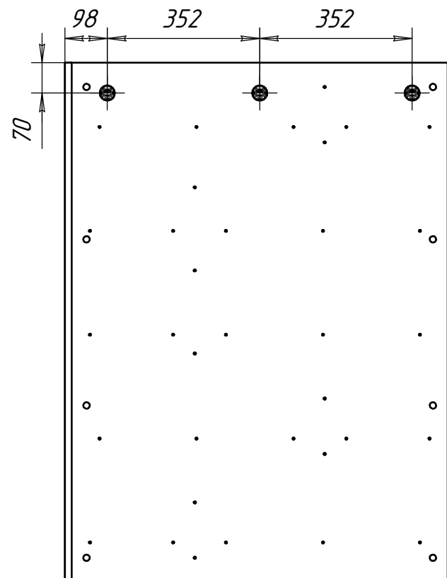
Схема полки 51.346.00.00 (вид сзади)
