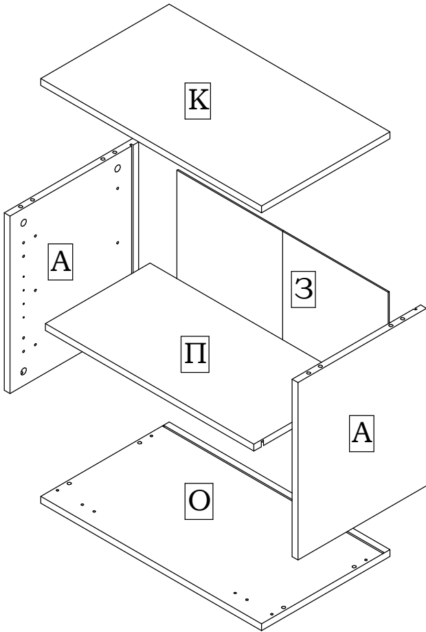
Комплект корпуса
