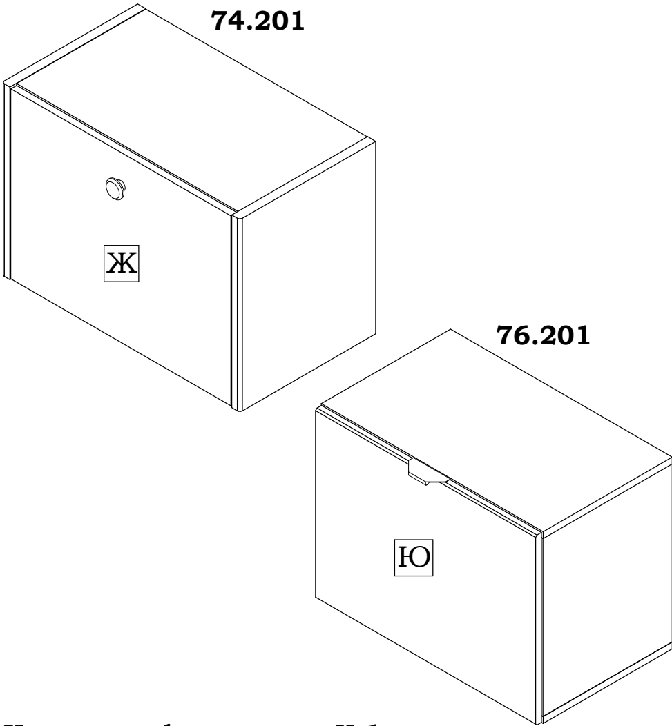
Комплект фурнитуры №1
