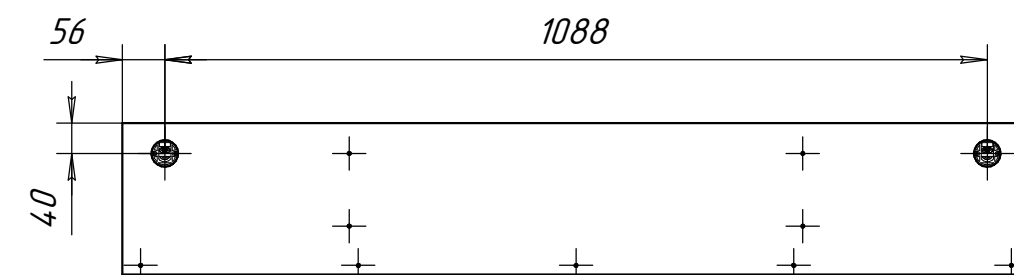
Схема полки 73.141.00.00 (вид сзади)
